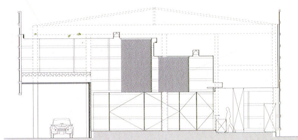
剖面图 1
