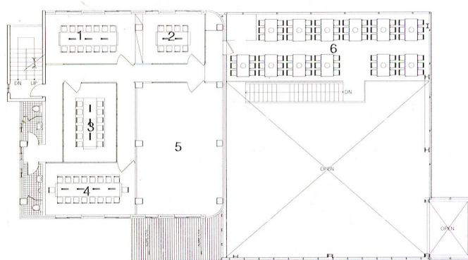
二层平面图
