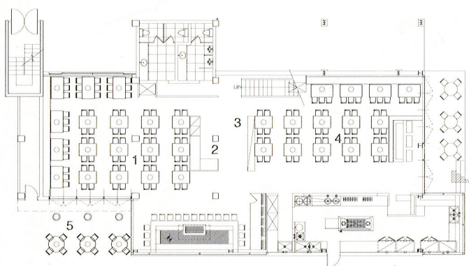
一层平面图
