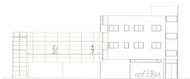
右侧面图
