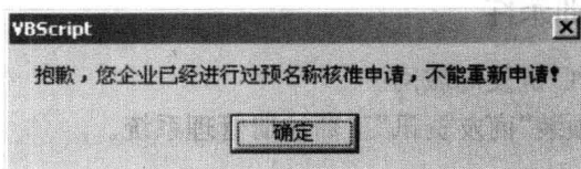
图 1.3 系统提示
