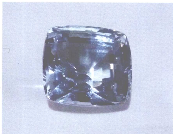
◀ 彩图 13 海蓝宝石
