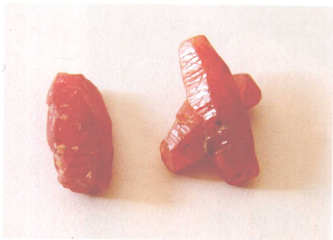
彩图 3 红刚玉晶体
