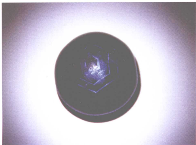
◄ 彩图 8 蓝宝石环带构造 (产地: 山东)
