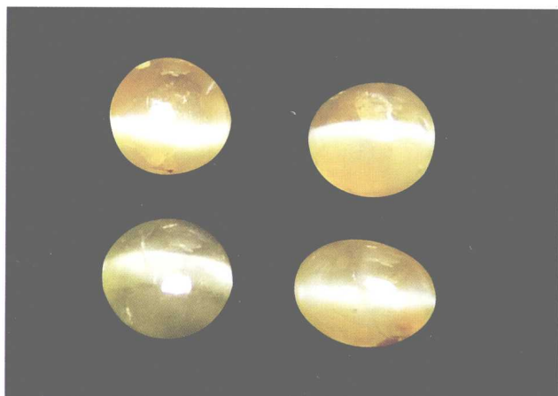
◀ 彩图 15 金绿猫眼
