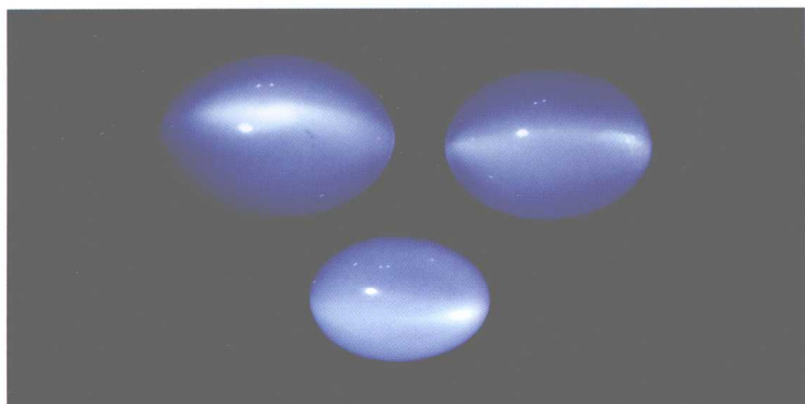
▲ 彩图 37 月光石 (猫眼效应)
