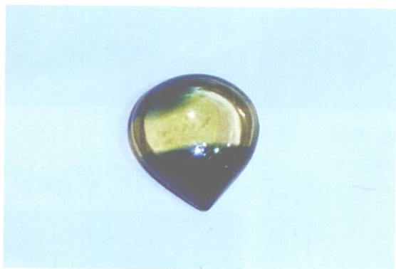
彩图 4 黄色蓝宝石 (产地: 山东)
