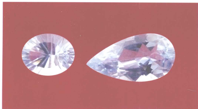
▶ 彩图 14 海蓝宝石
