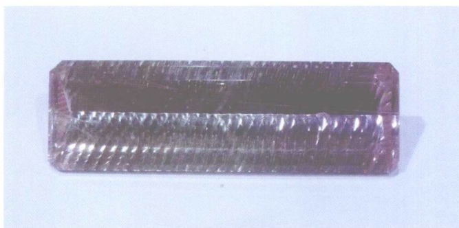
▲ 彩图 41 紫锂辉石
