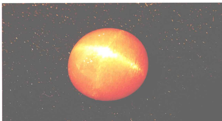
▲ 彩图 38 日光石 (十字星光)
