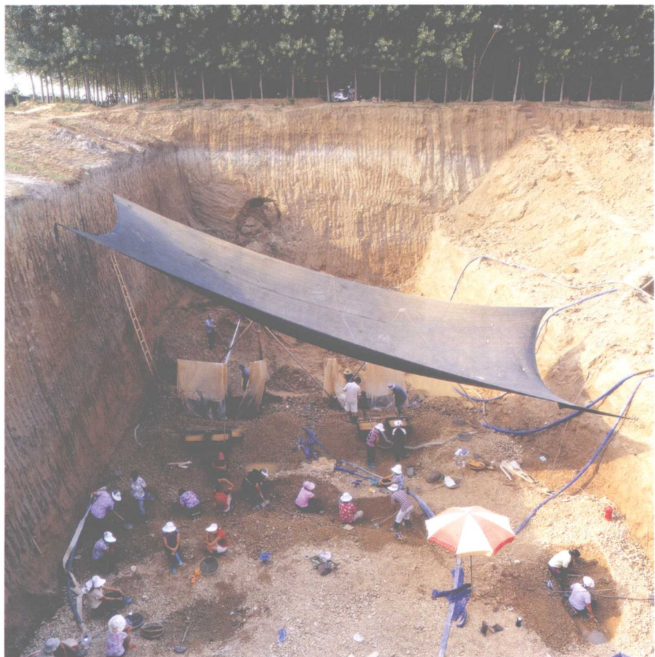
▲ 彩图9 蓝宝石砂矿采矿现场 (山东)
