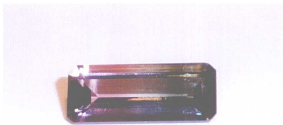
彩图 20 多色碧玺 (产地: 新疆)
