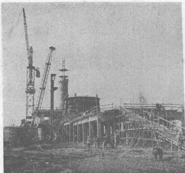
← 武鋼一號高爐開始吊裝出鐵場鋼制柱子。
