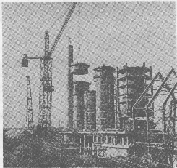
→ 武鋼一號高爐在吊裝熱風爐外殼。
