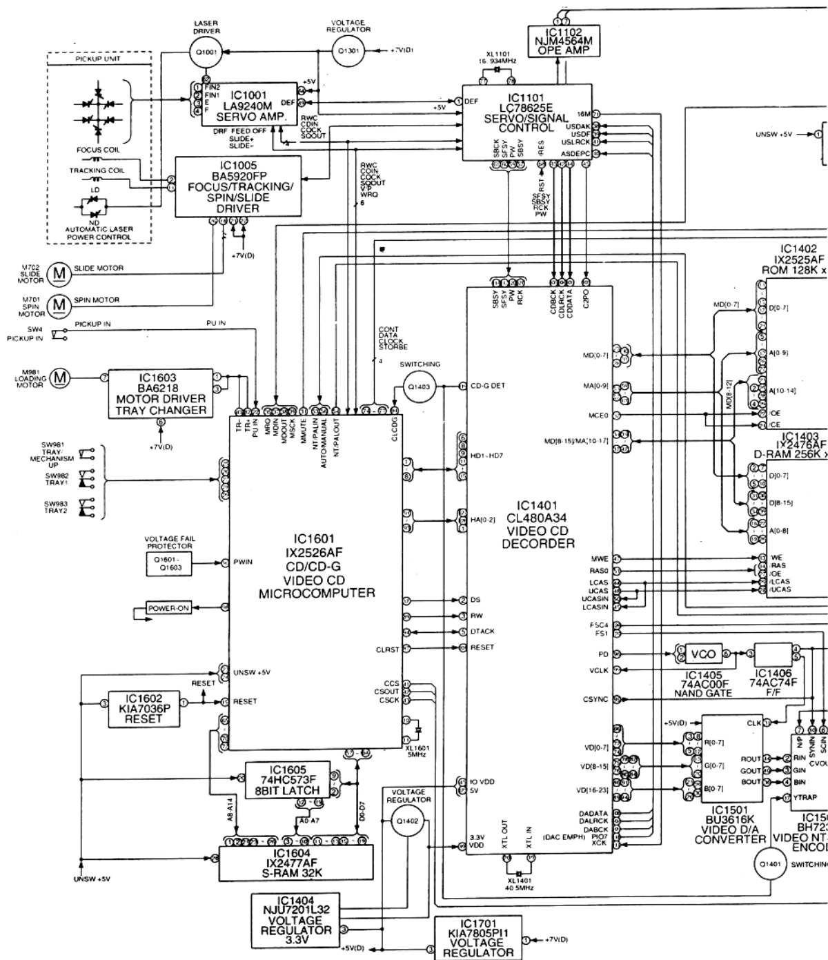
夏普 DX-V200X 型激光影碟机方框图(1)
