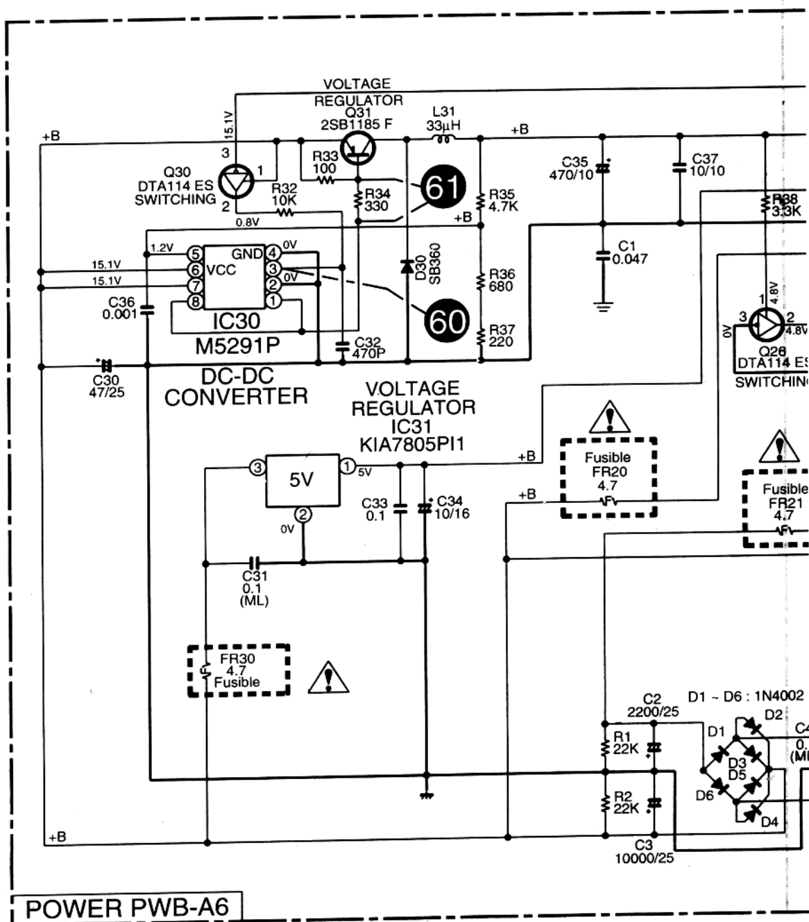
夏普 DX-V200X 型激光影碟机电路图(7)
