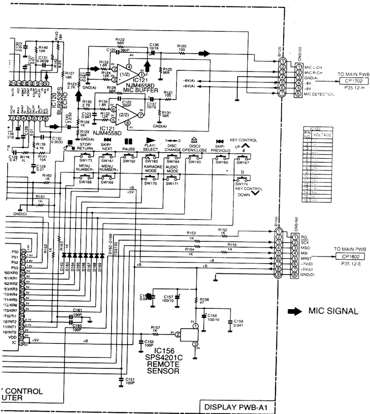
夏普 DX-V200X 型激光影碟机电路图(6)
