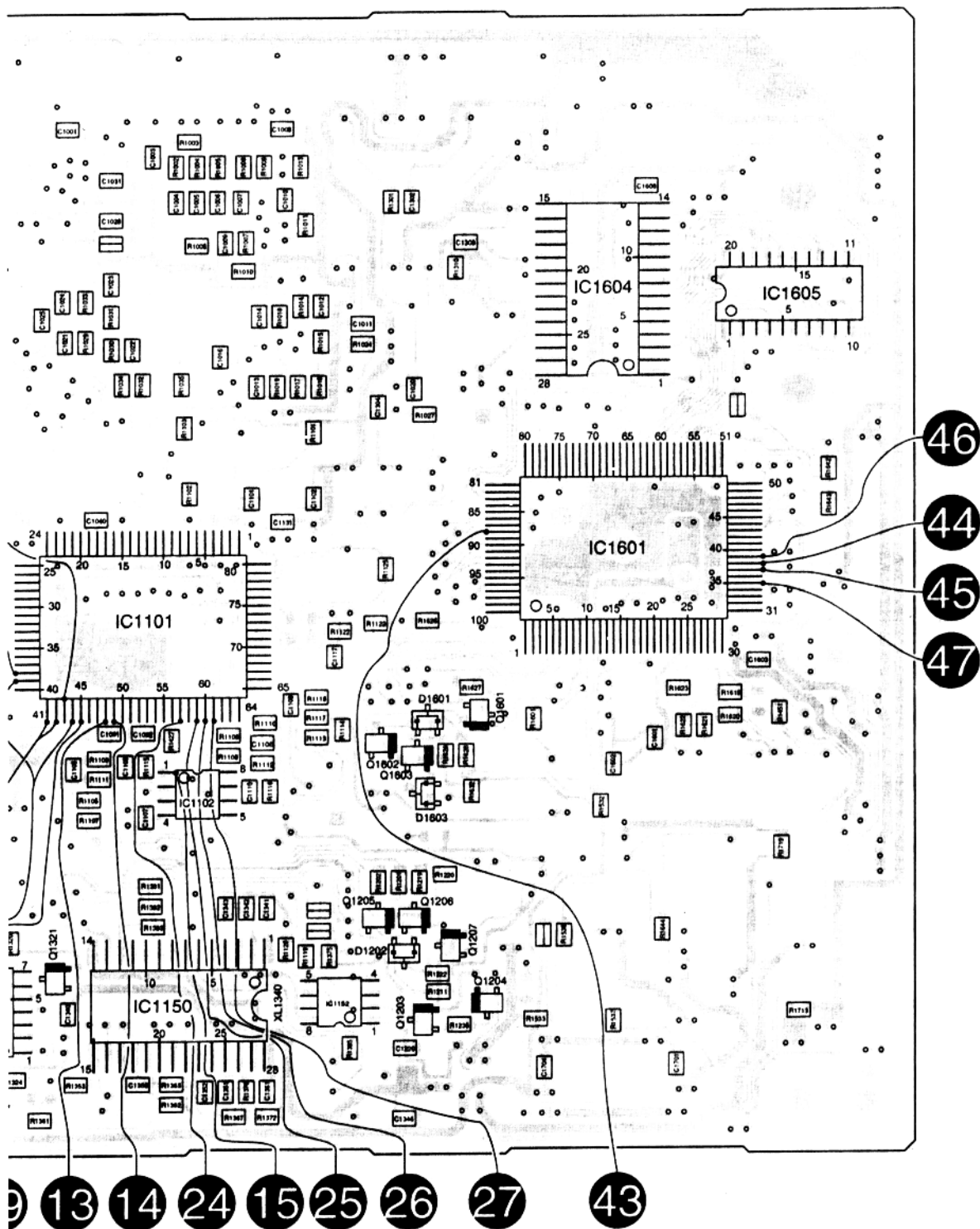
夏普 DX-V200X 型激光影碟机印刷板图(2)
