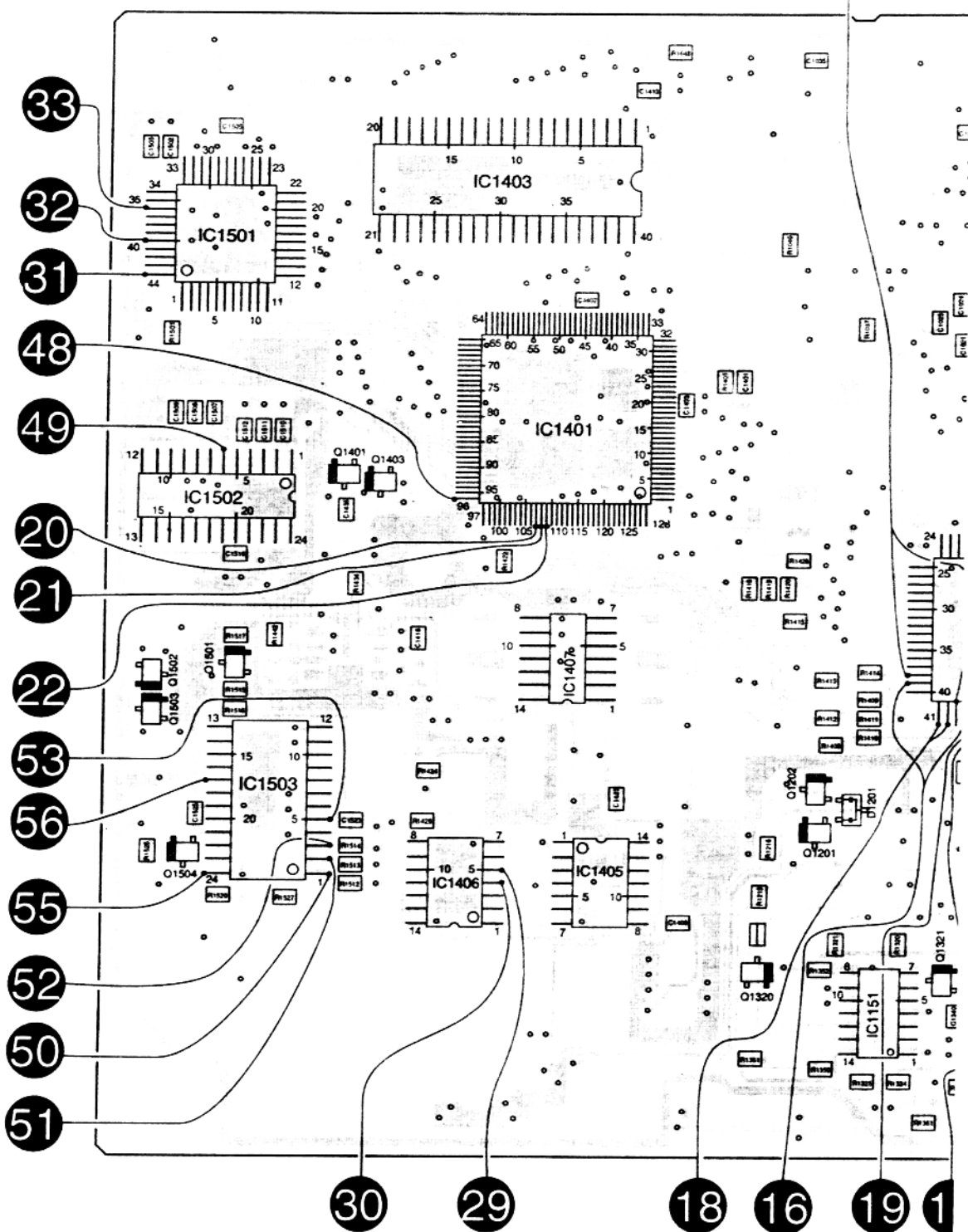
夏普 DX-V200X 型激光影碟机印刷板图(1)
