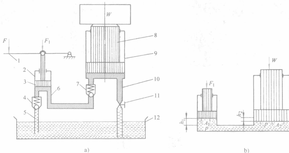
图 0-1 液压千斤顶
