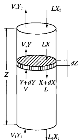
图 1-1 微元填料层的物料衡算
