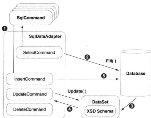
图2 用 SqlDataAdapter 更改数据
