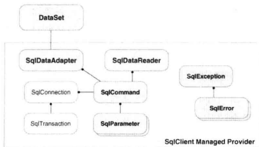
图 1 SqlClient 对象模型
