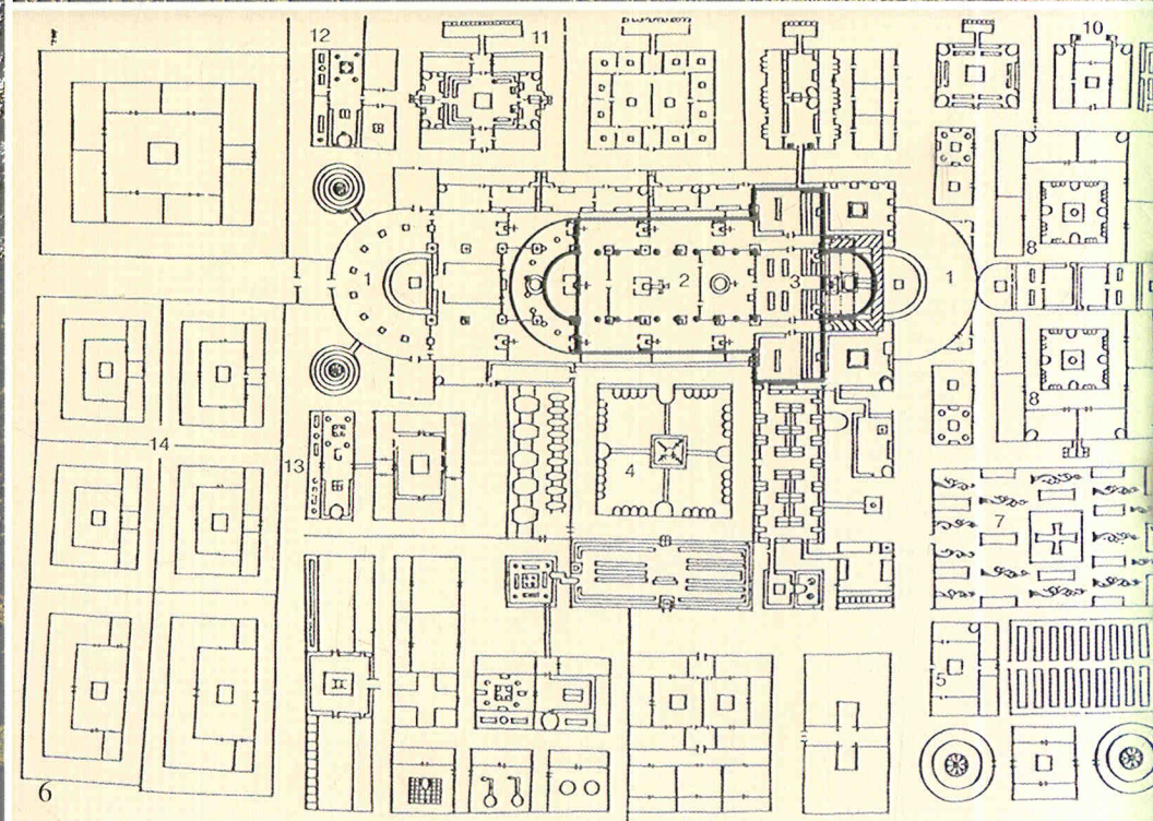
6. 圣戈尔修道院(ST. GALL MONASTERY) 公元 820 年建造 布局图: 1、前院 2、教堂正厅 3、合唱厅 4、回廊 5、园丁住所 6、菜园 7、墓地 8、见习修士学校和医院 9、药草园 10、诊所和药物存放所 11、客厅 12、帐房 13、酒窖与面包房 14、马厩。
