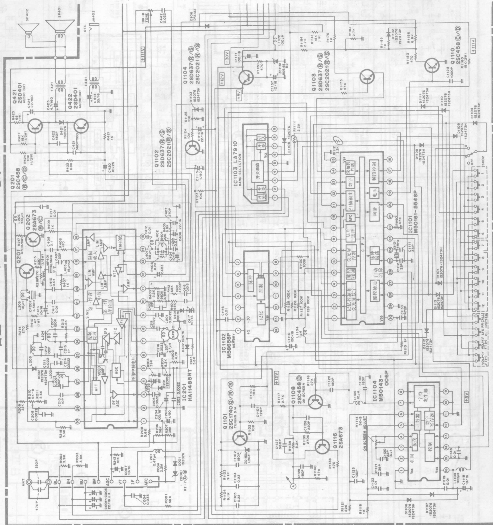
日立NP84C20/CPT-2005 电原理图
