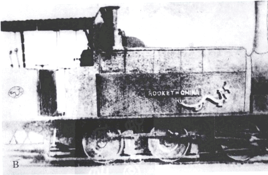
20.A.B.开平矿务局自制的中国最早的机车及龙号机车
