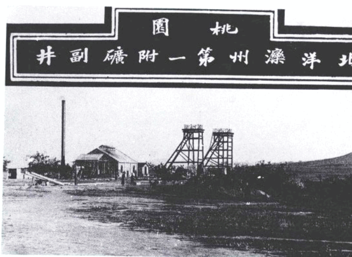
22.北洋滦州官矿有限公司 陈家岭矿桃园副井
