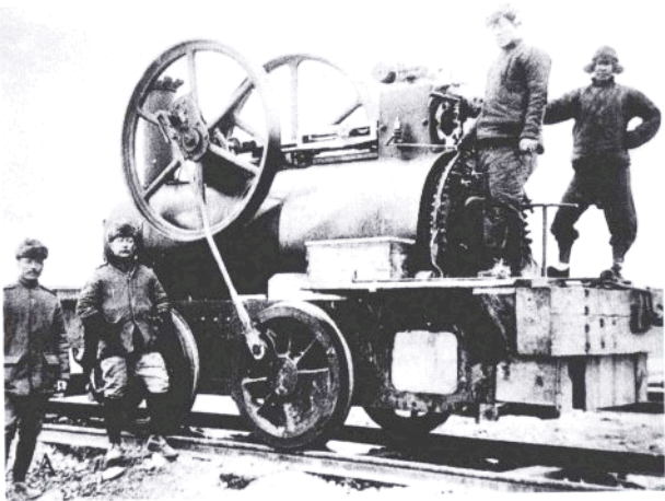
20.A.B.开平矿务局自制的中国最早的机车及龙号机车
