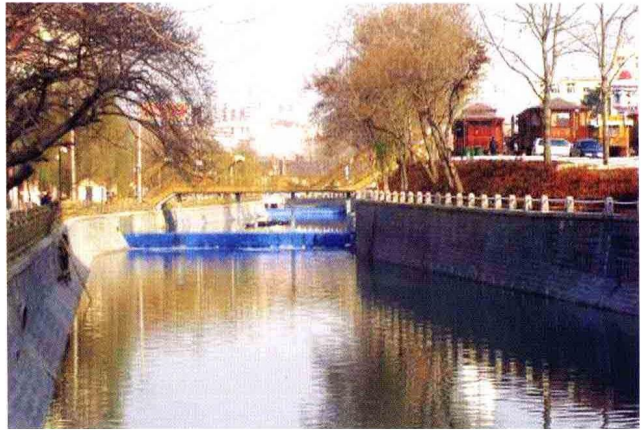
海泊河河道中密集的橡胶坝
