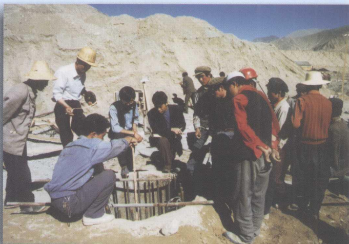
▶ 钢筋笼位置检测
