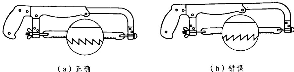
图 1.11 锯条的安装方法
