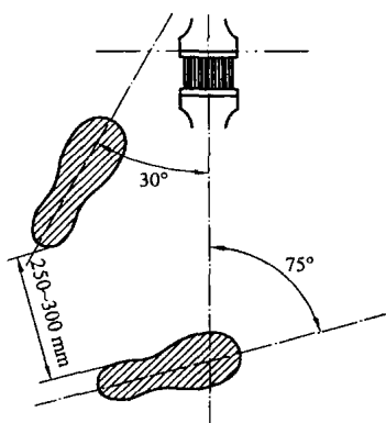
图 1.5 鍬削工件时的站立位置
