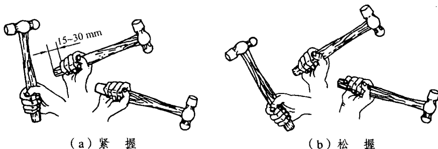
图 1.2 手锤的握法
