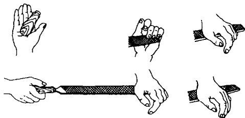
图 1.7 板锉的握法
