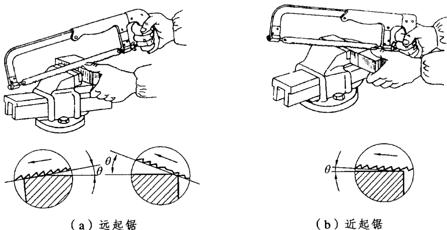
图 1.12 起 锯
