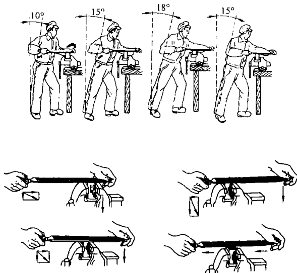
图 1.9 锉削姿势
