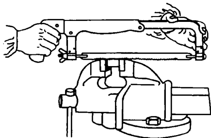
图 1.10 手锯握法
