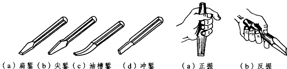
图 1.3 鍬 子
