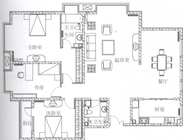
平面布置图
