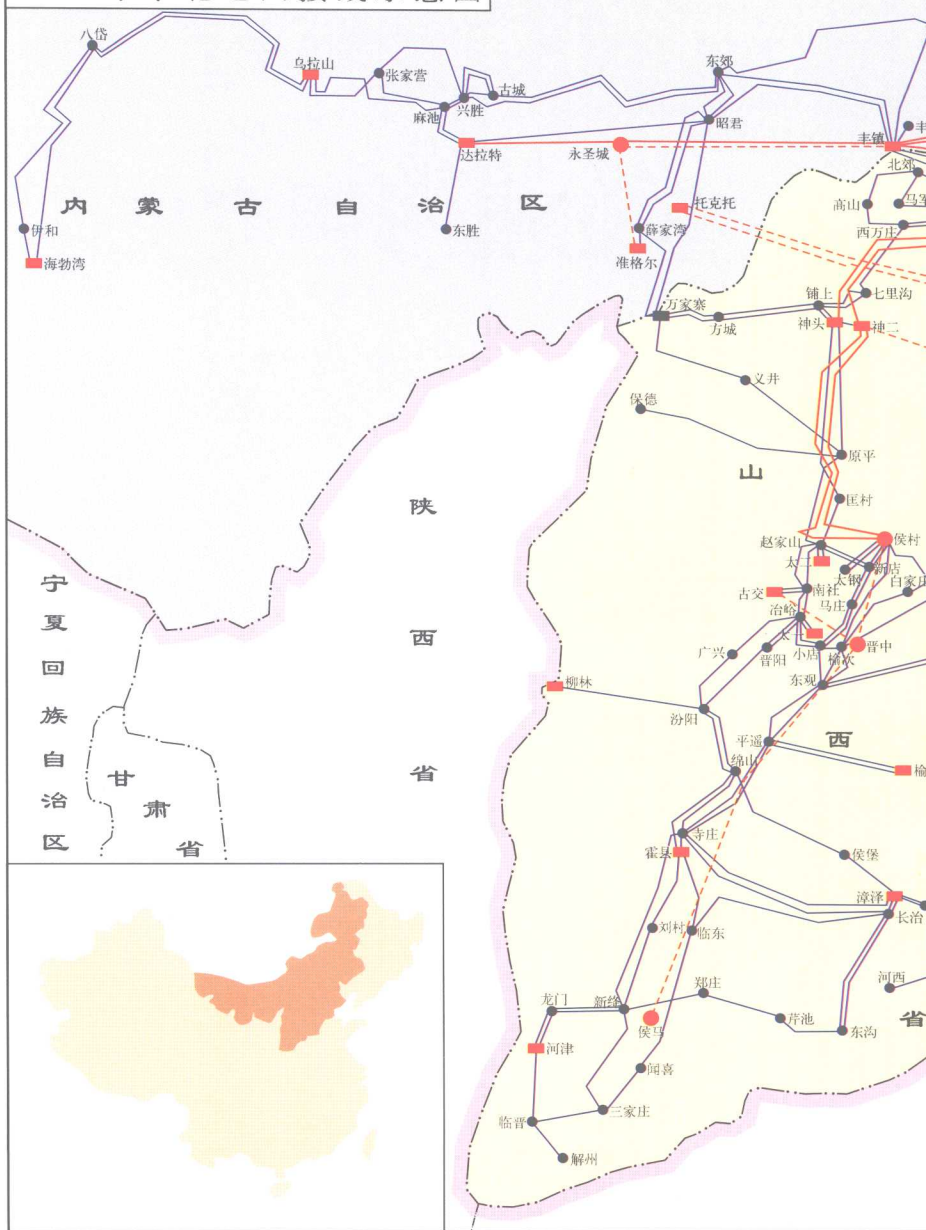
1999年华北电网接线示意图
