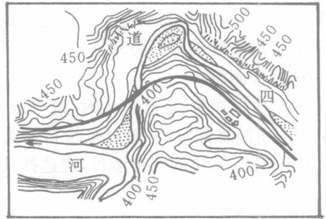
图 2-3 “S”形河段中部跨河线形
