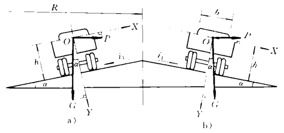
图 2-7 汽车在曲线上行驶的横向力 a)内侧;b)外侧
