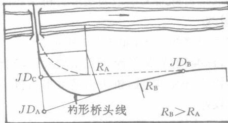
图 2-6 桥头杓形布线
