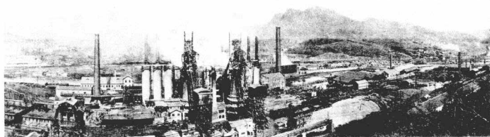
本溪湖煤铁公司工厂全景（1930年）
