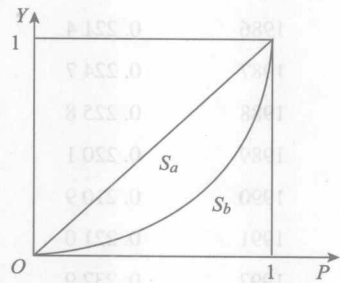
图1 洛伦兹曲线图
