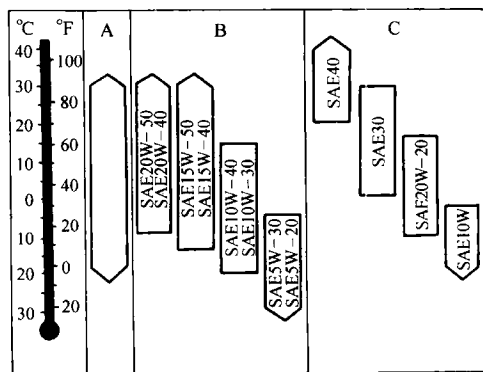
图 1—8 发动机机油适用的温度范围
