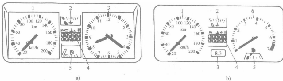
图 1—2 组合仪表构造
