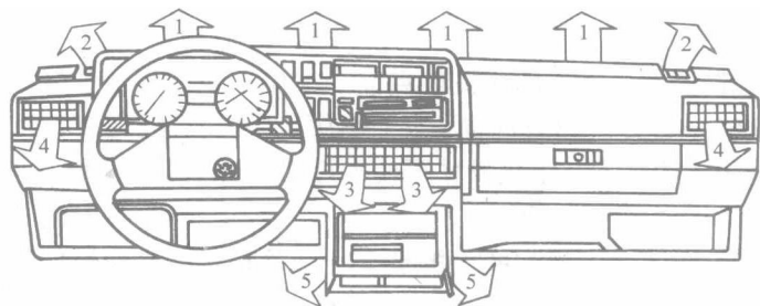
图 1—6 空调器出风口的布局
