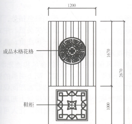
鞋柜立面图
