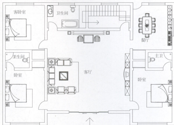
一层平面布置图
