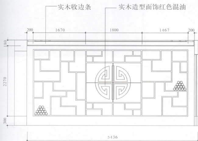
书柜施工图
