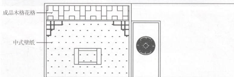
电视背景墙立面图
