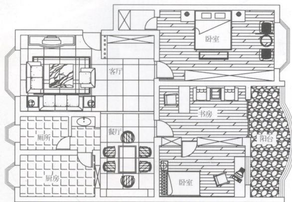
平面布置图
