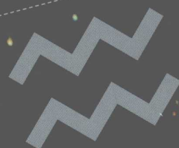
Aquarius
