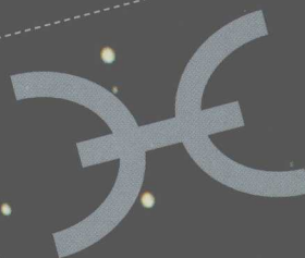
Pisces
