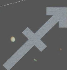
Sagittarius
