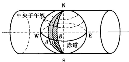
图 1.7 高斯平面直角坐标的投影
