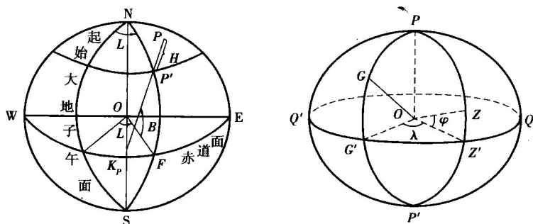
图 1.4 地理坐标系
