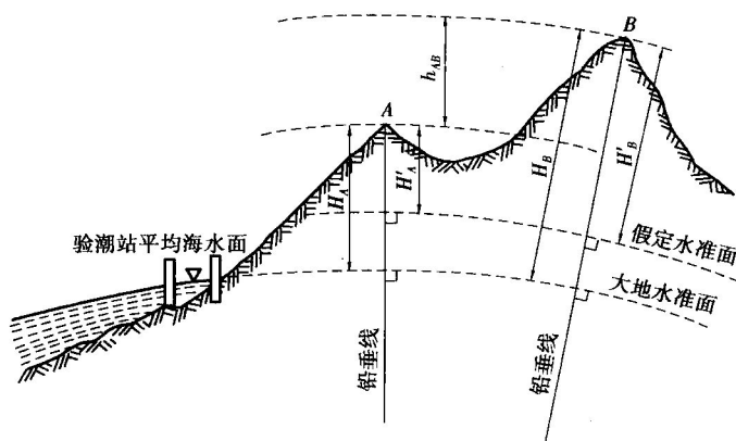
图 1.10 高程系统
