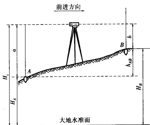
图2.1 水准测量基本原理
