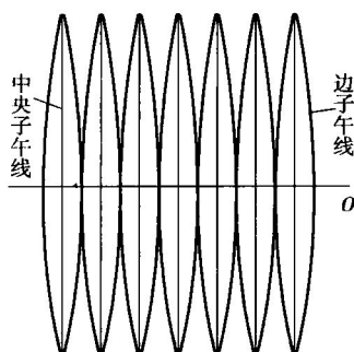
图 1.6 高斯分布带
