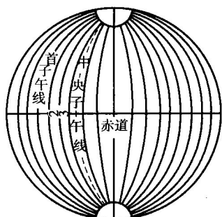
图 1.5 高斯投影
