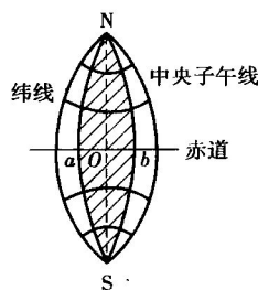
图 1.6 高斯分布带
