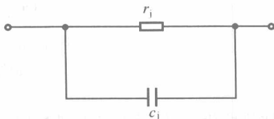
图 1-7 PN 结高频等效电路
