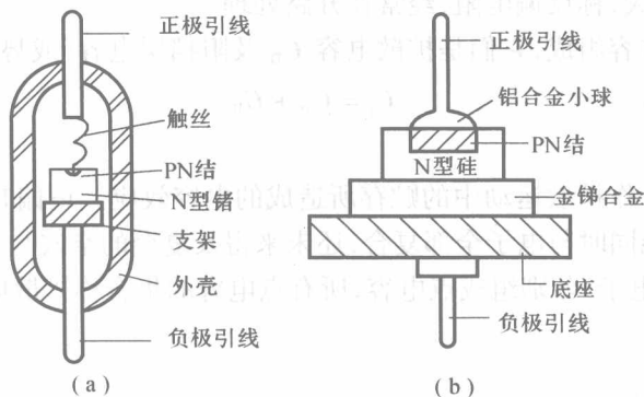
图 1-9 二极管的结构
