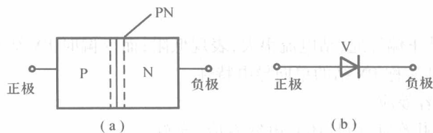
图 1-8 二极管的结构示意图与电路符号
