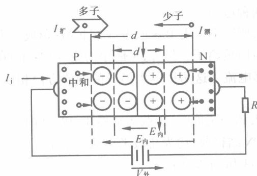
图 1-5 PN 结正向加压
