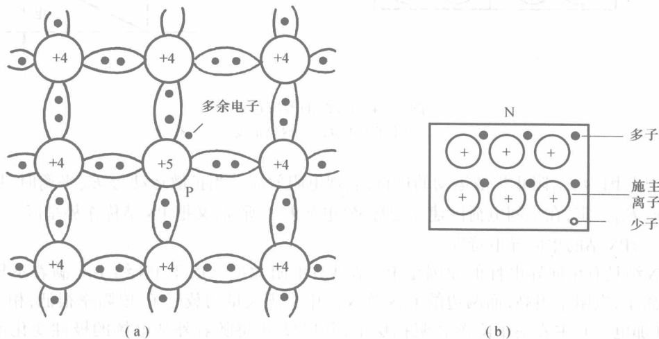
图1-3 N型半导体中的载流子
