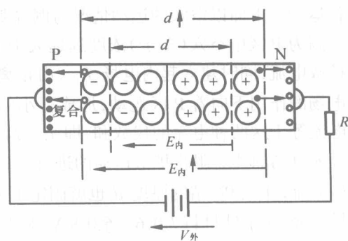
图 1-6 PN 结反向加压
