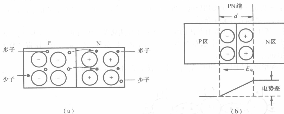
图 1-4 PN 结的形成过程
