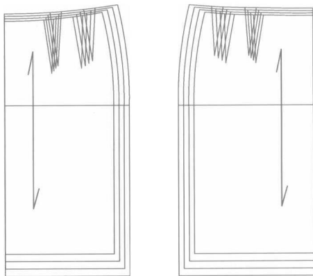
图1-4 直身裙网状推档图
