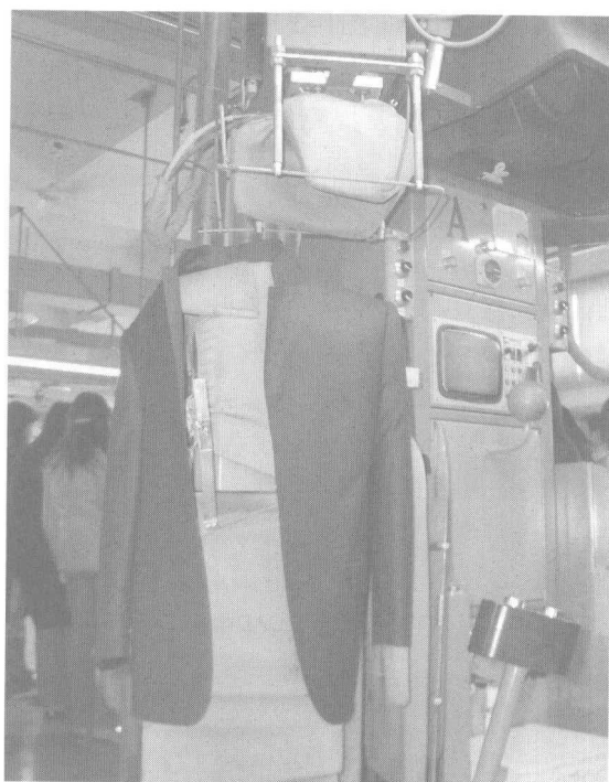
图1-6 立体整烫机
