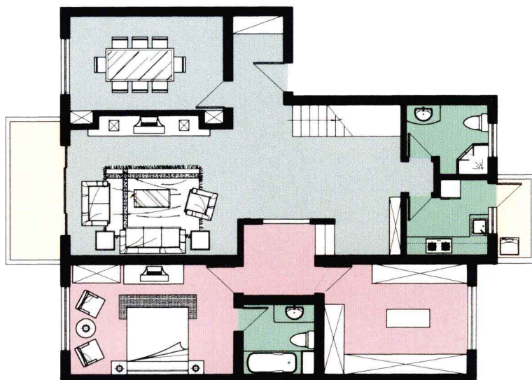
一层现状平面图
