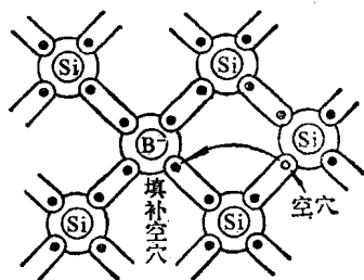
图 8-8 硅晶体中掺硼出现空穴
