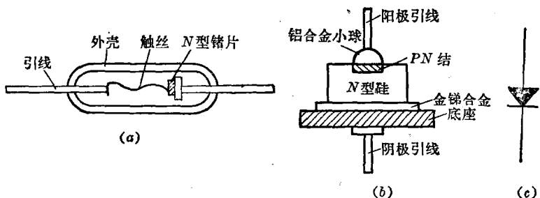
图 8-13 半导体二极管:
