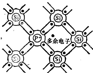
图 8-6 硅晶体中掺磷出现自由电子
