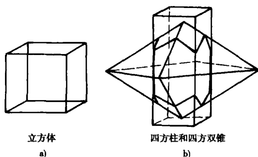
图 1-1 a) 单形; b) 聚形
