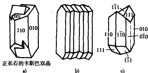
图 1-3 几种双晶类型
