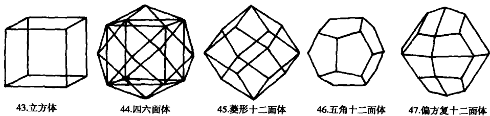
图 1-2 矿物晶体的 47 种单形
