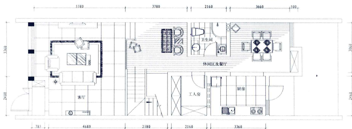
一层平面布置图
