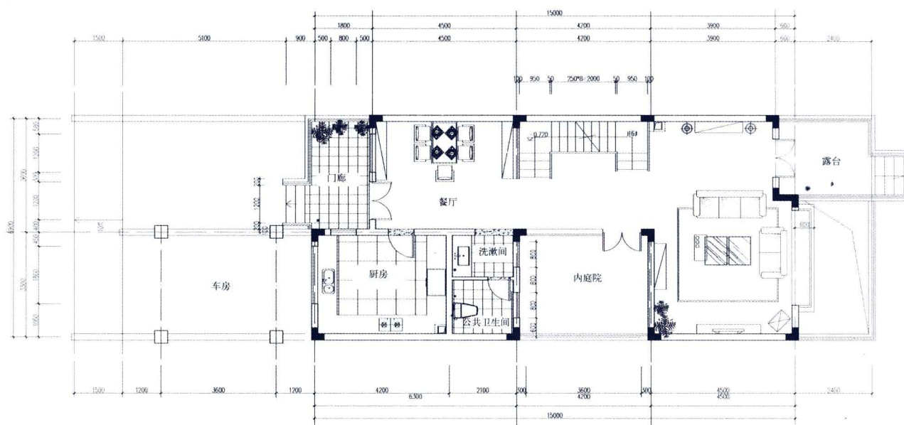
一层平面布置图
