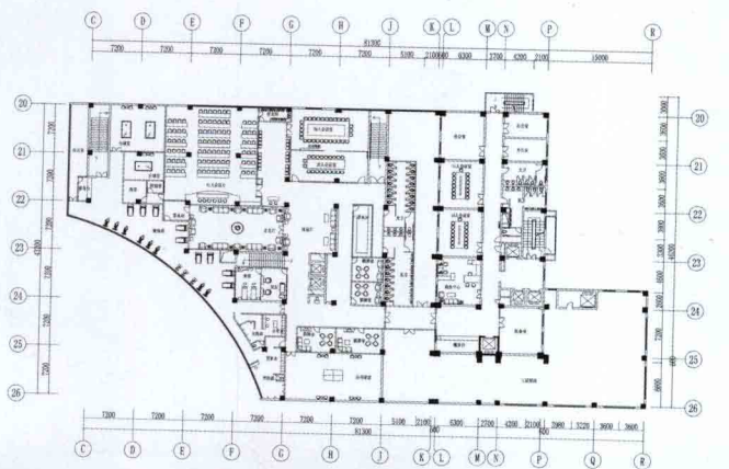
四层平面图
