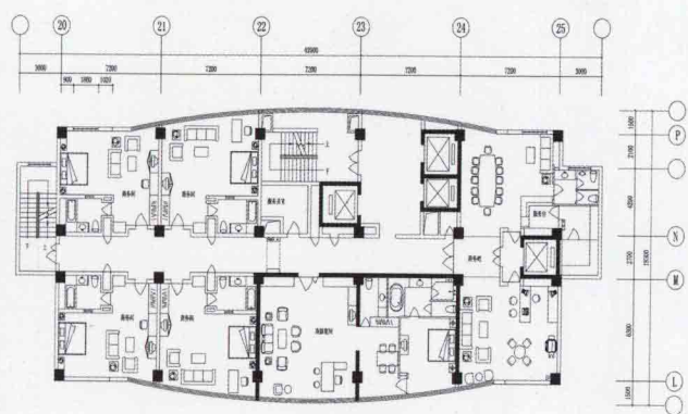
六~八层平面
