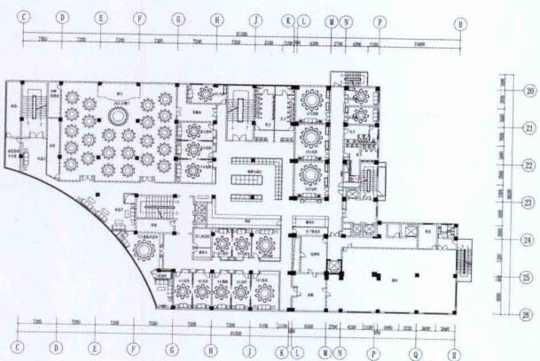
二层平面图
