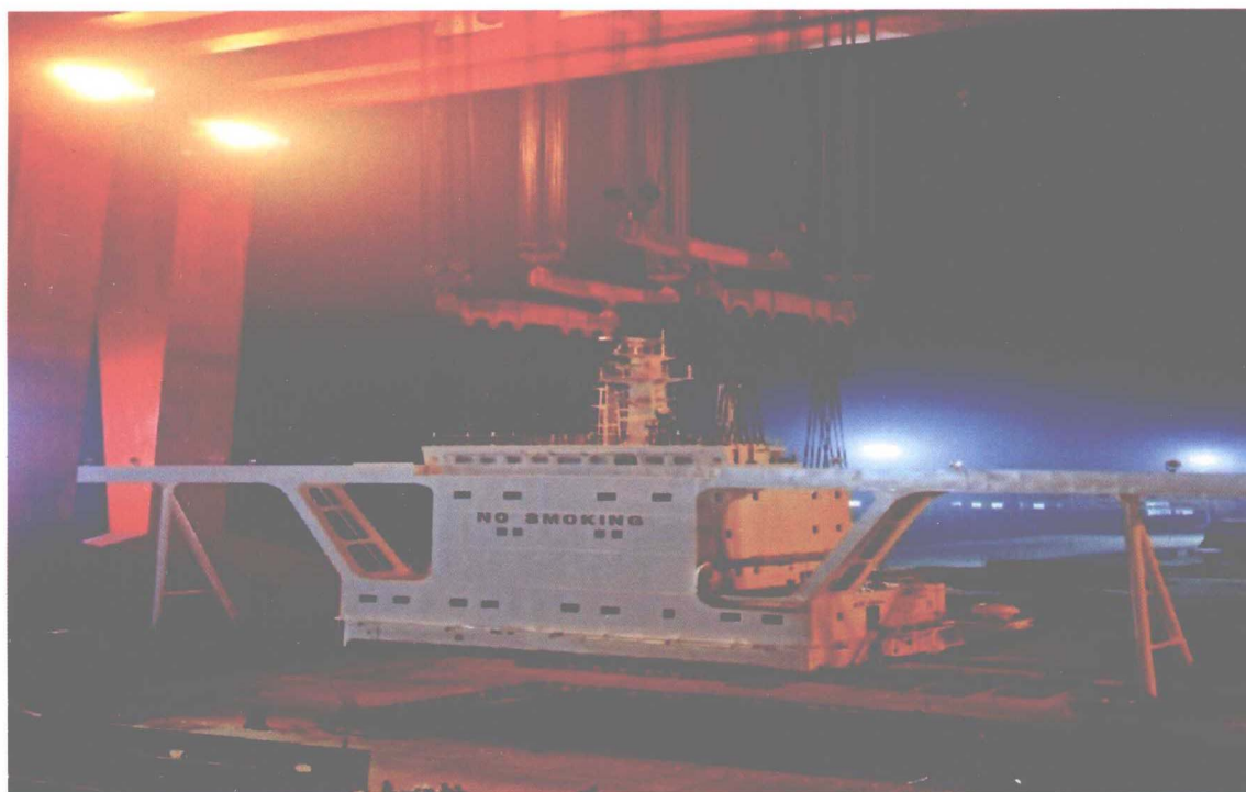
公司大型上层建筑模块正在进行吊装
