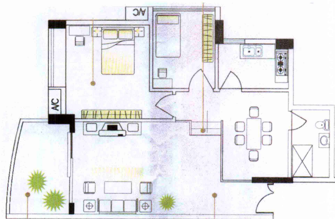
■ 广州柏涛雅苑 79.95 平方米户型图
