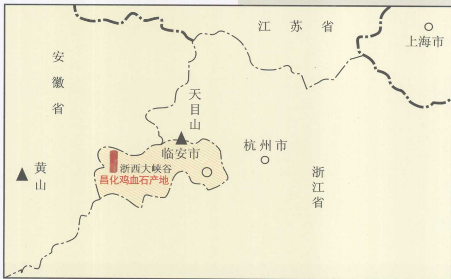
昌化鸡血石矿地理位置图
