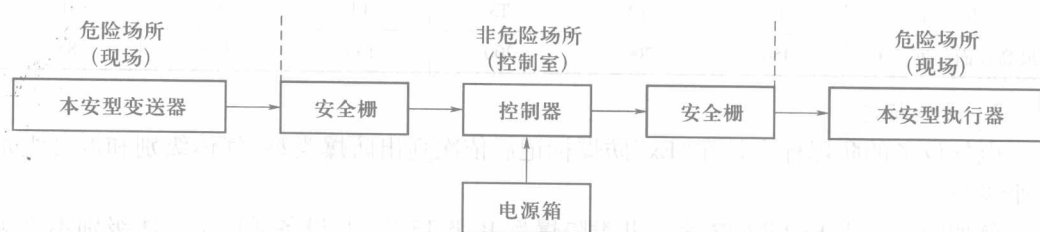
图 1-6 本安防爆系统
