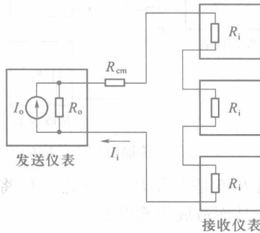
图 1-2 电流信号传输时仪表之间的连接
