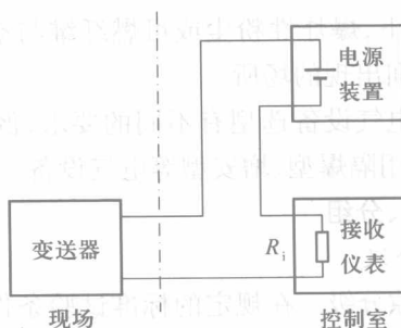
图 1-5 两线制传输
