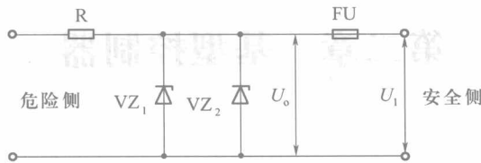
图 1-7 齐纳式安全栅
