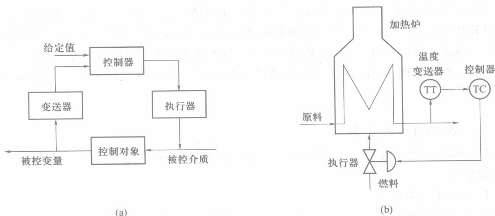
图 1-1 控制系统简图
