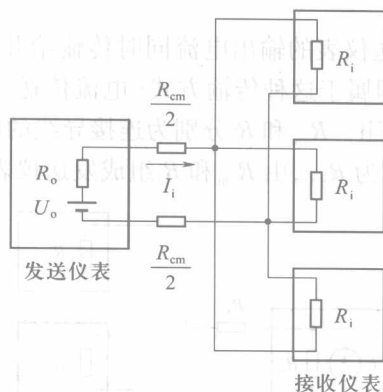
图 1-3 电压信号传输时仪表之间的连接
