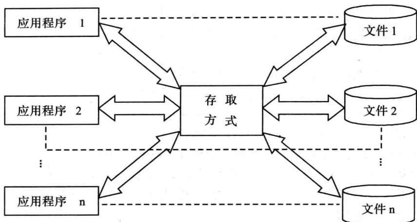
图 1—3 文件系统阶段应用程序与数据之间的对应关系
