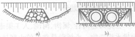
图 1-3 透水路堤
