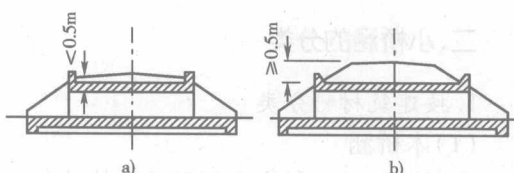
图 1-6 涵洞按填土高度分类
