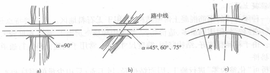
图 1-10 小桥涵按洞身平面布置分类
