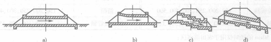
图 1-9 涵洞按洞身形式分类
