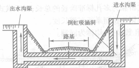
图 1-4 倒虹吸涵洞
