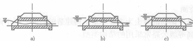
图 1-8 涵洞按水力性质分类
