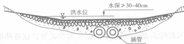
图 1-2 过水路面
