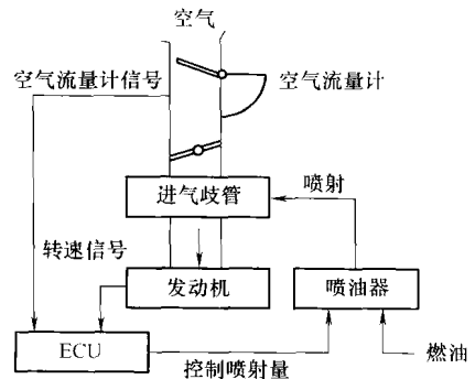
图 2-3 L型电控燃油喷射系统基本工作原理
