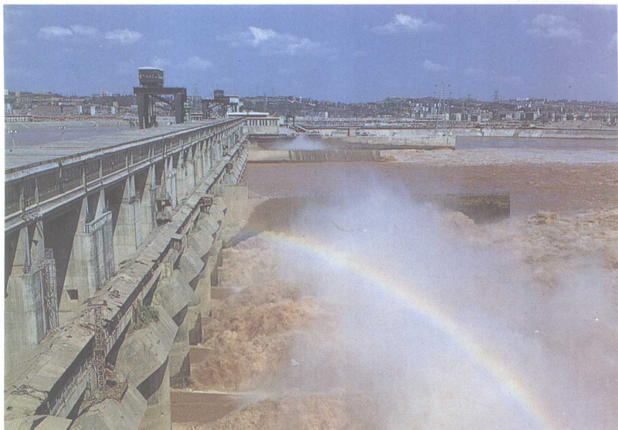
葛洲坝雄姿
