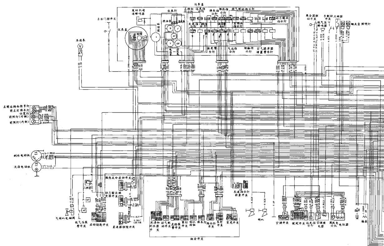
图3 三菱 (MITSUBISHI) FP、FU、FV 型全气制动载重汽车电路图 (a)
