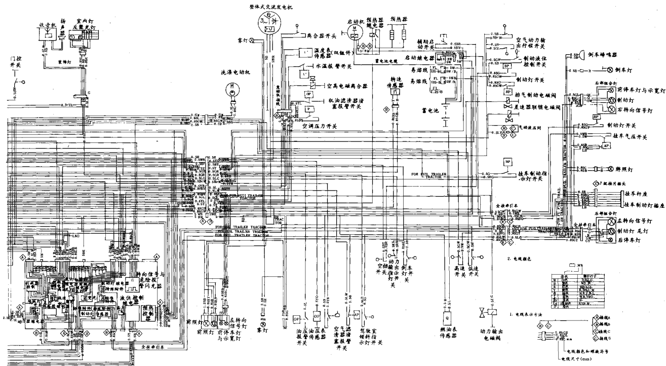
图2 三菱扶桑（FUSO）FP、FU、FV气、液压制动重型载货汽车电路图（b）
