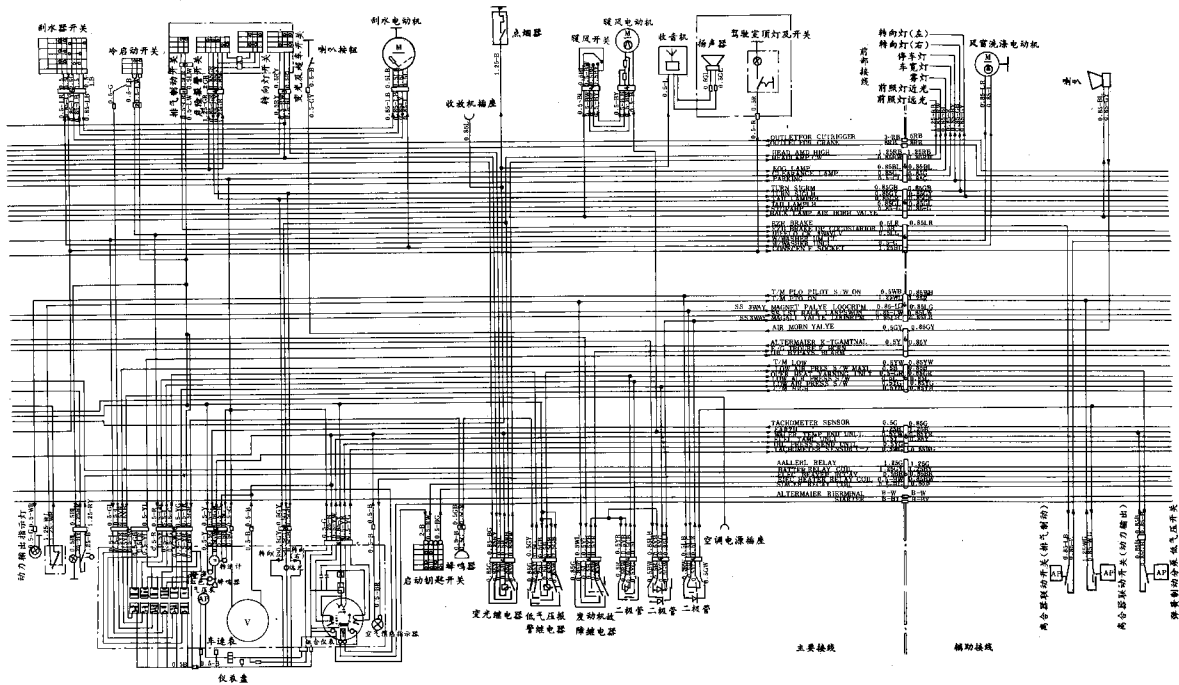
图5 三菱扶桑 (FUSO) K402 型底盘电路图 (b)
