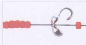
①将串珠线的末端穿入线夹，并接着穿入1颗小米珠。
