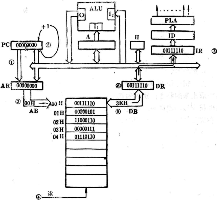
图1-7 取第一条指令的操作示意图
