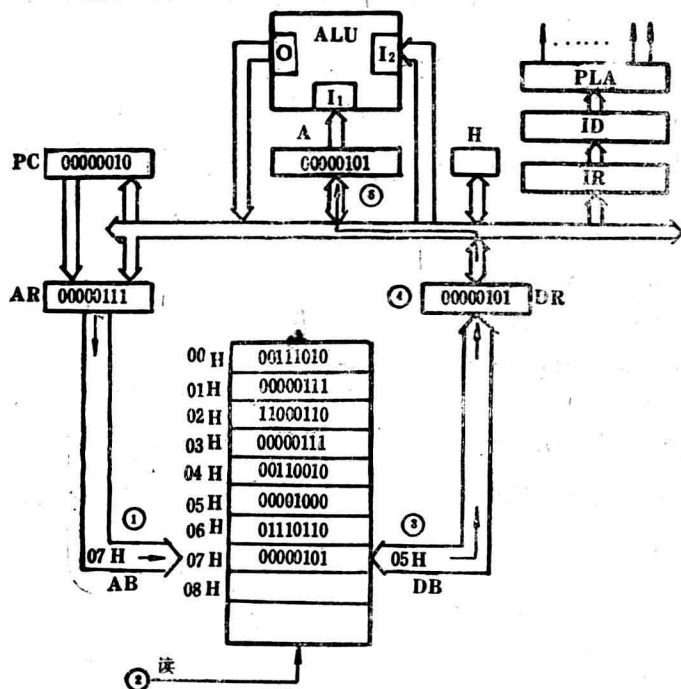
图1-15 取操作数的操作示意图
