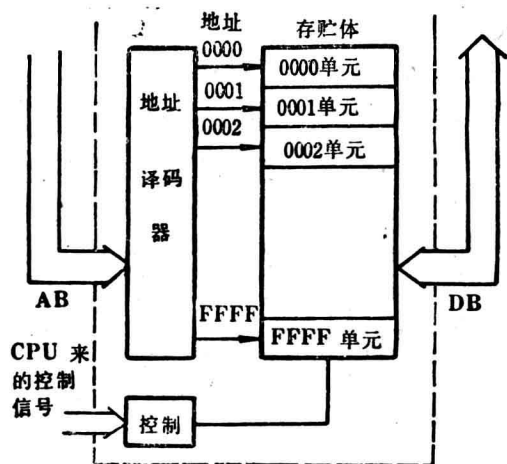
图1-2 存储器结构图
