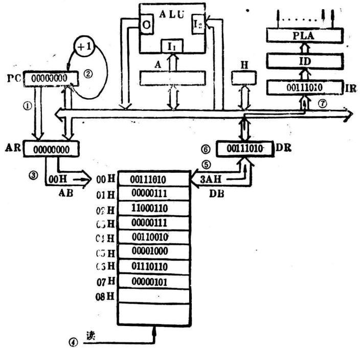
图1-13 取第一条指令的操作示意图
