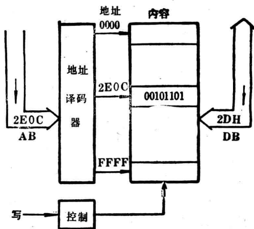
图1-4 存储器写操作示意图
