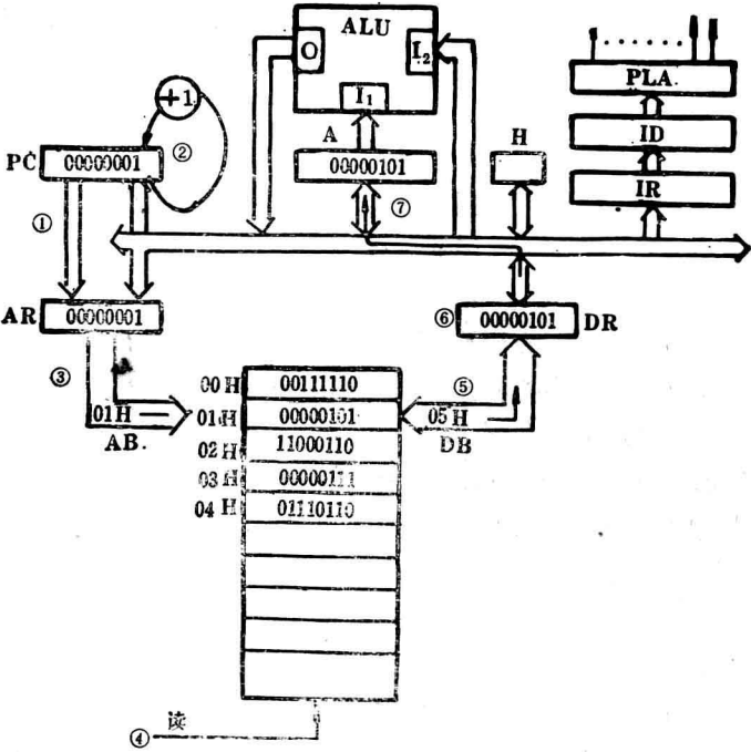
图1-8 执行第一条指令的操作示意图
