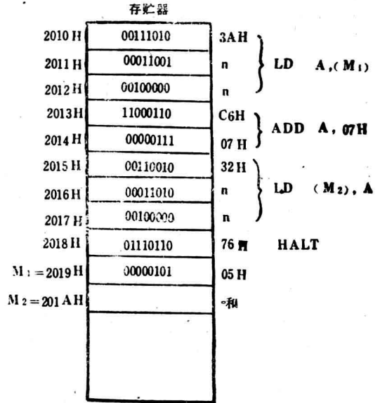
图1-16 程序存储示意图
