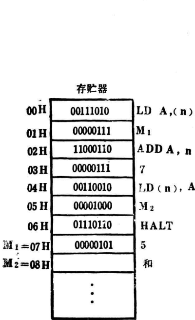
图1-12 程序存储示意图
