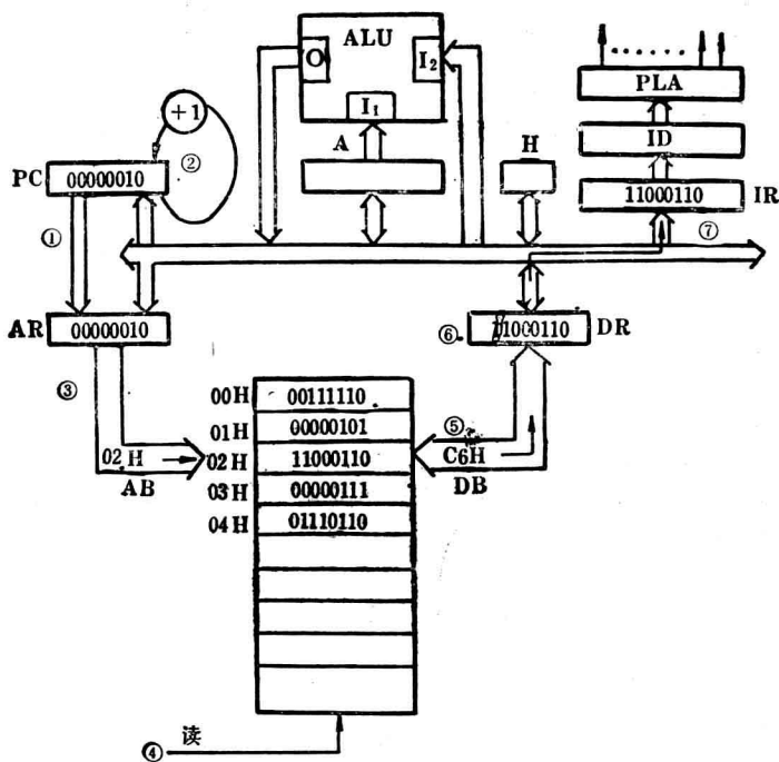
图1-9 取第二条指令操作示意图
