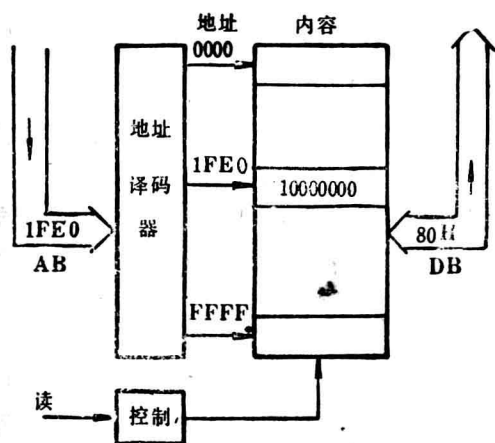
图1-3 存储器读操作示意图
