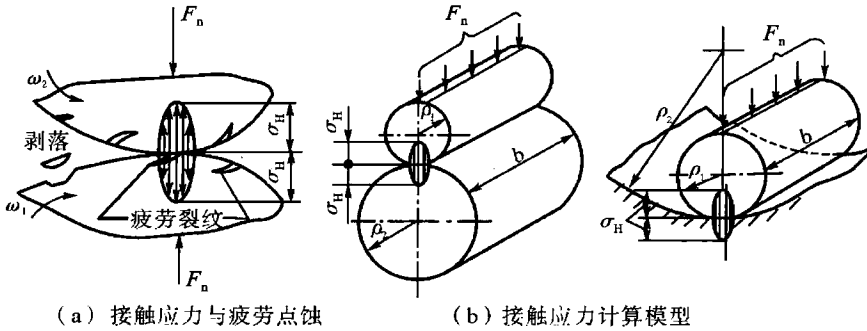
图 1-5 疲劳点蚀和接触应力计算模型
