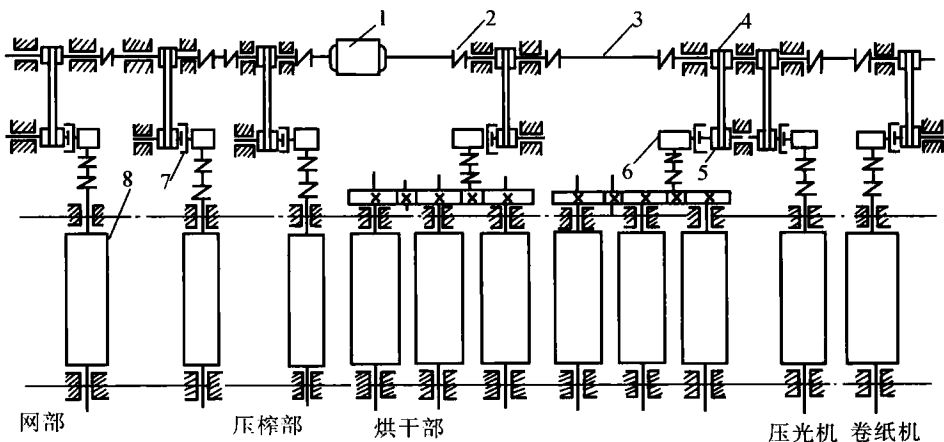
图 1-1 造纸机简图
