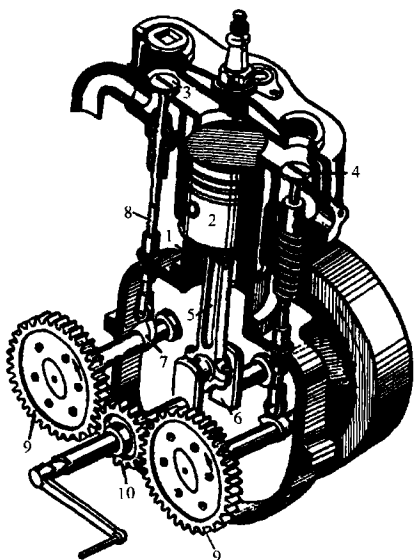
图 1-2 内燃机
