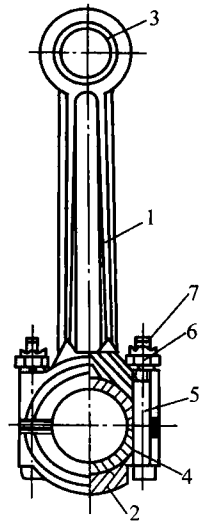
图1-4 连杆
