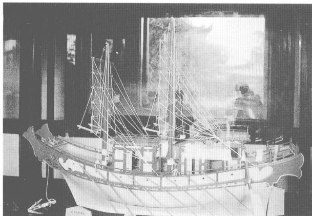
唐天宝年间鉴真和尚东渡日本船舶（船模）
