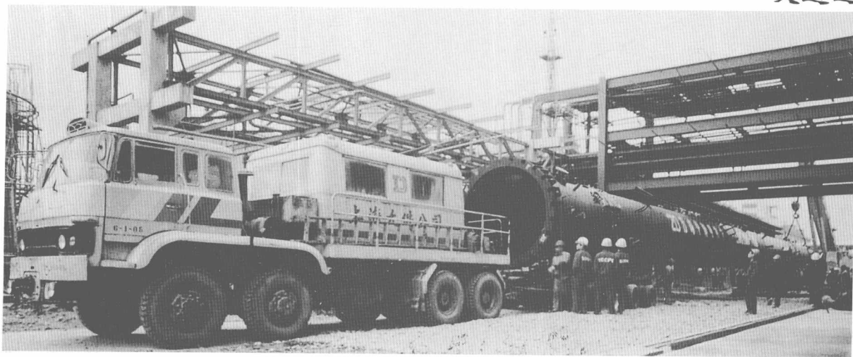
大型设备运抵安装工地
