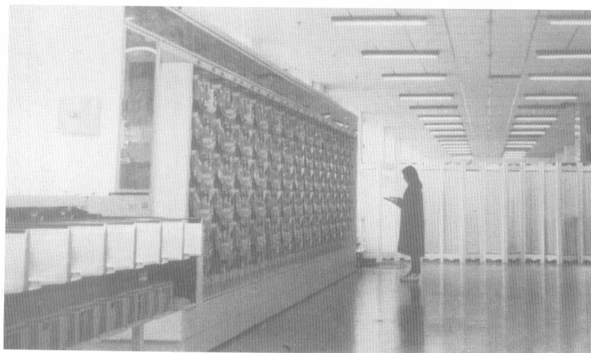
1992年向德国引进的AEG全自动出口信函分拣机及机房
