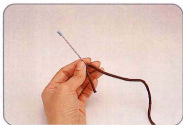
② 洞口太小时用的穿线器（洞口1cm用）。
