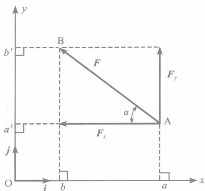
图 1-3 力的投影
