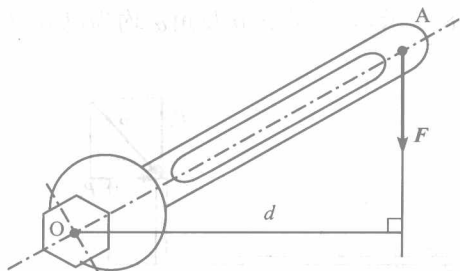
图 1-5 力的转动效应
