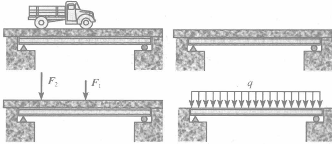
图 1-1 集中力与分布力
