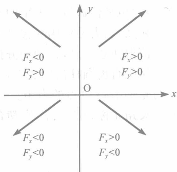
图 1-4 投影符号和力指向的关系
