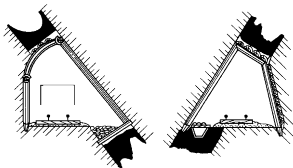
图 2-7 不规则形状的巷道
