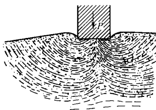
图 1-5 木块压沙试验
