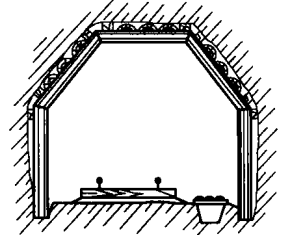
图 2-4 多角形巷道
