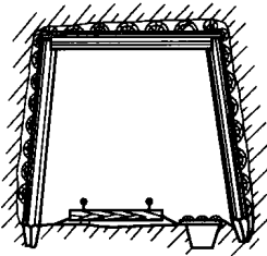
图 2-3 梯形巷道
