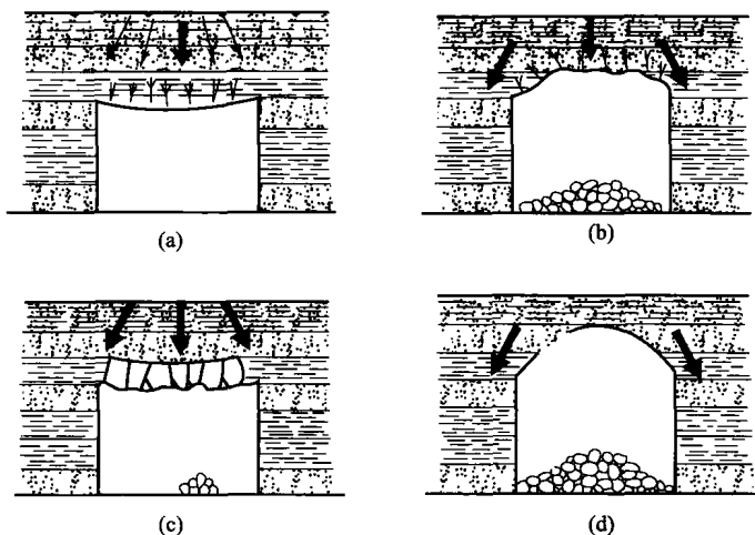
图 1-3 巷道顶压的产生
