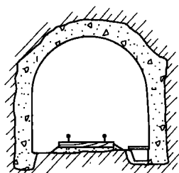
图 2-5 拱形巷道
