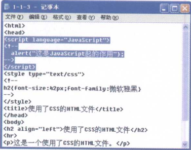
图0-2 代码环境——记事本
