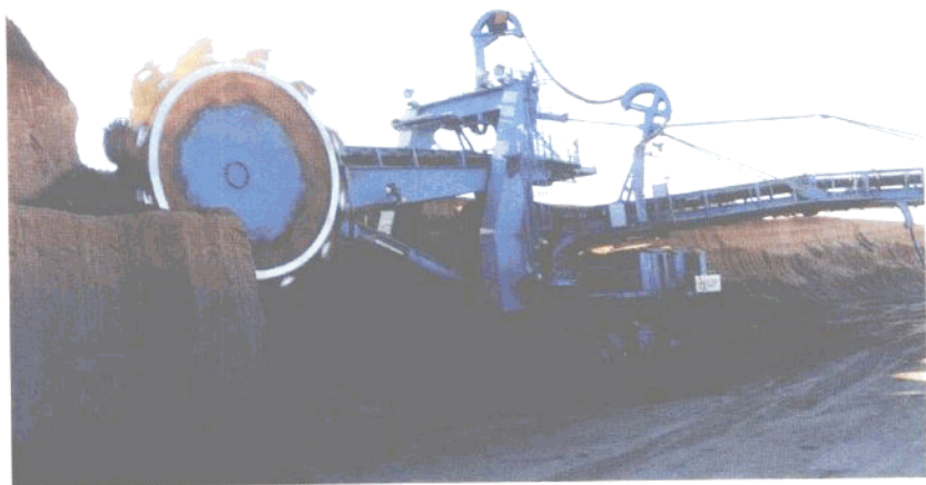
国家重点建设工程——准格尔煤田表土分离
