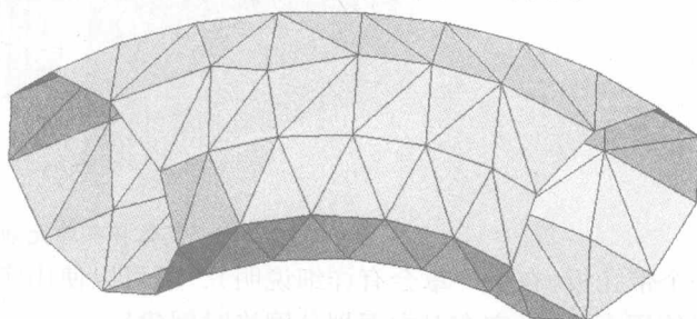
图 0-8 一阶三角形壳单元网格划分结果
