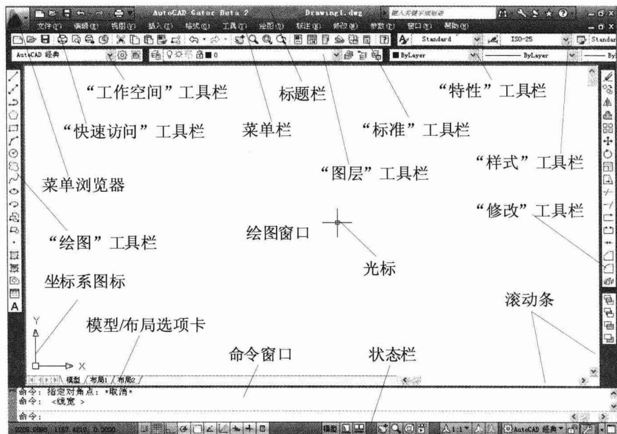
图 1-1 AutoCAD 2010 经典工作界面
